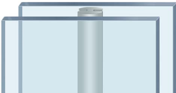
Alu-Sprosse im Glaszwischenraum, 2-fach Verglasung
