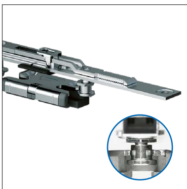
Sicherheitsverriegelungsstelle
